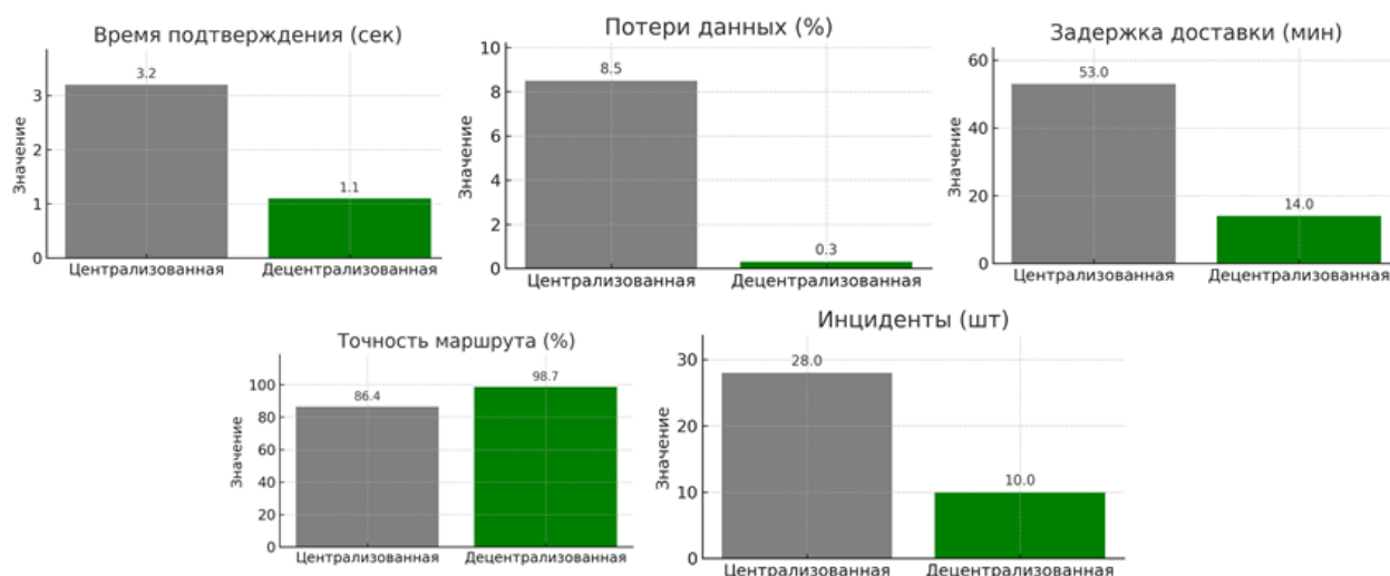
Рисунок 2 - Сравнение централизованной и децентрализованной модели по ключевым метрикам
