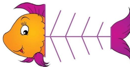
Рисунок 2 – Фишбоун
