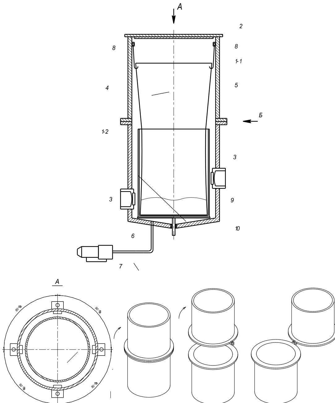
Рисунок 1 – Установка для вакуумной СВЧ – сушки и обработки материалов
