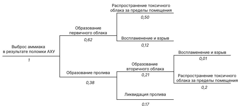
Рисунок 3 – Дерево событий поломки аммиачной холодильной установки
