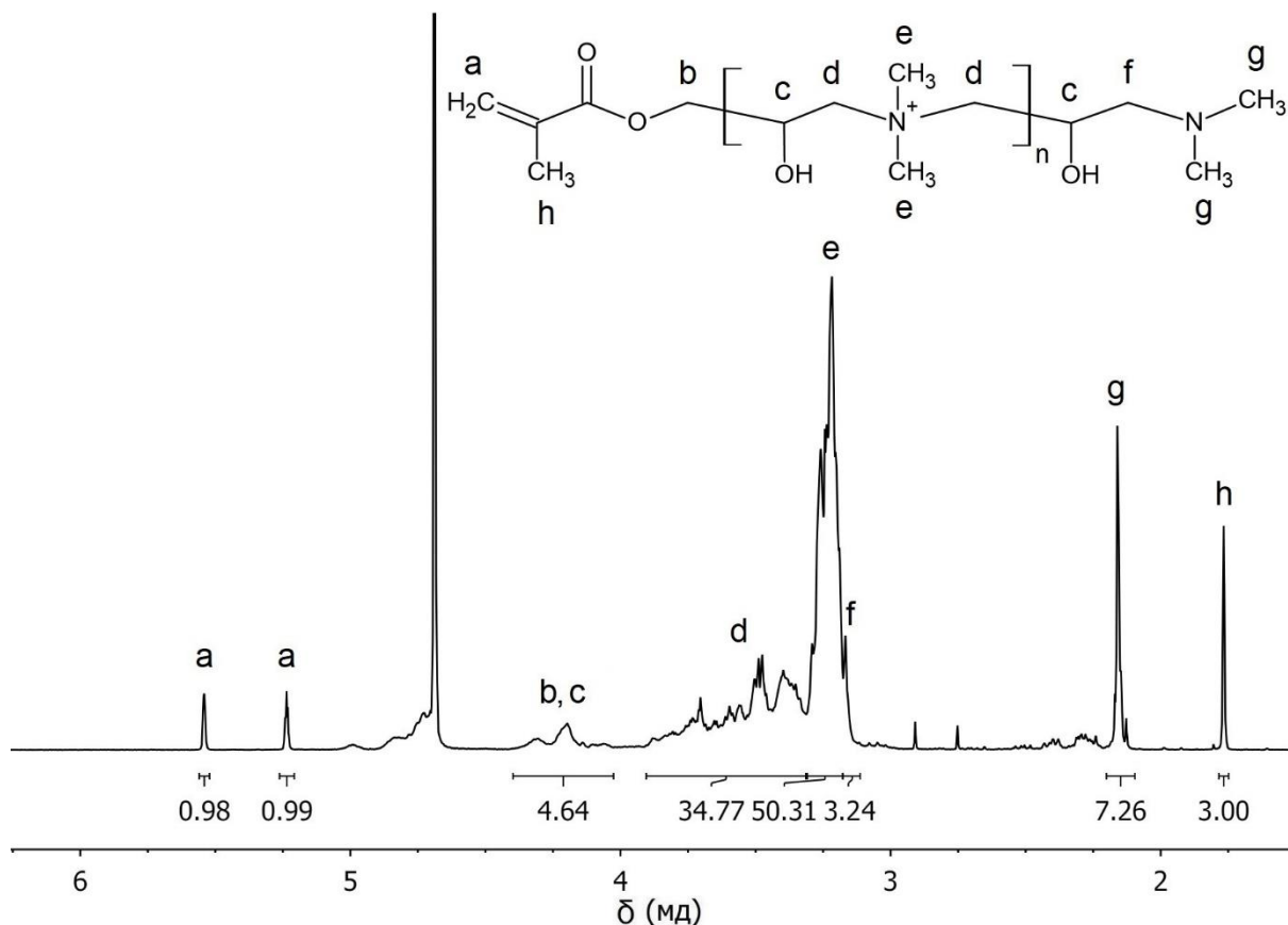
Рисунок 3 – ПМР-спектр макромономера, растворитель D 2 O
