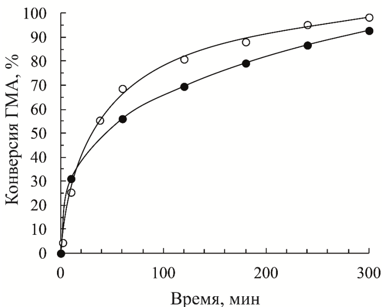
Рисунок 2 – Конверсия ГМА при мольном соотношении [ЭХГ]: [БДАП]: [ГМА] = 5:5:1 (○), [ЭХГ]: [БДАП]: [ГМА] = 2,6:2,6:1 (●). Температура синтеза 15 °С.
