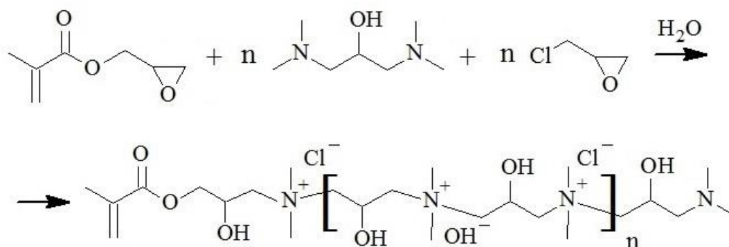
Рисунок 1 – Синтез макромономера поликонденсацией ЭХГ и БДАП в присутствии ГМА
