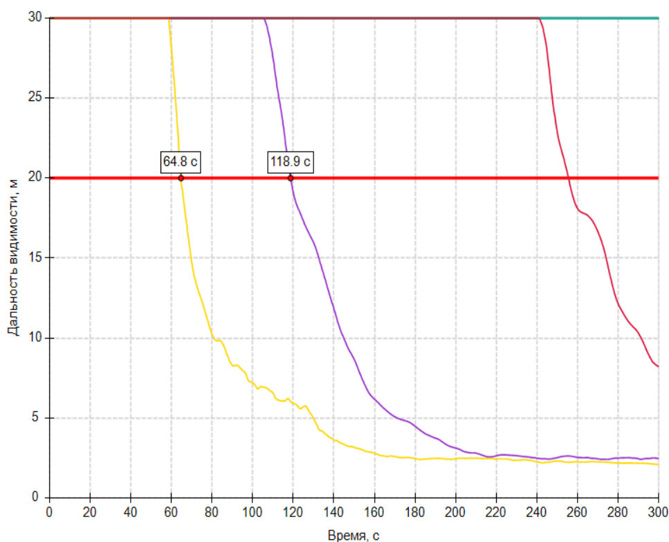
Рисунок 2 – Время достижения критических значений дальности видимости
