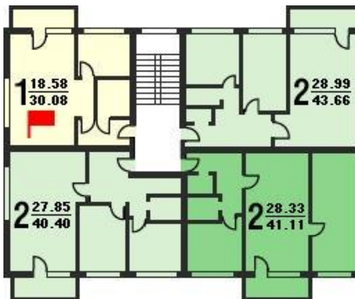
Рисунок 1 – Планировка типового этажа
