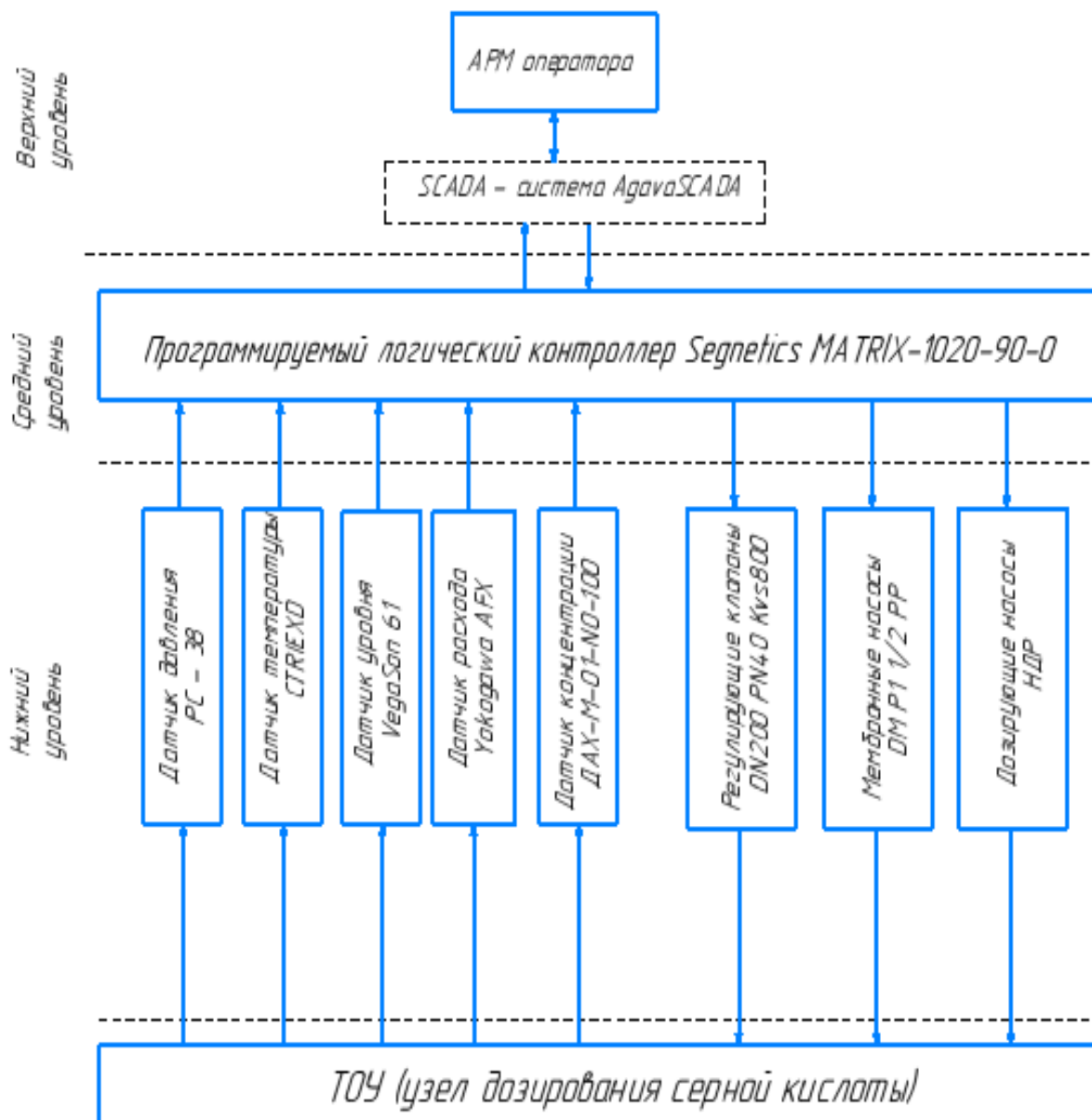
Рисунок 1 – АСУ узлом дозирования серной кислоты
