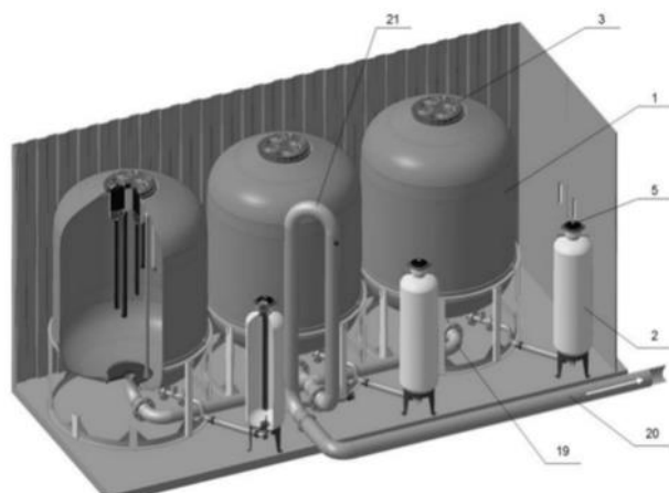
Рисунок 2 – Схема устройства модуля пожаротушения с генератором давления (МППД) [3]
