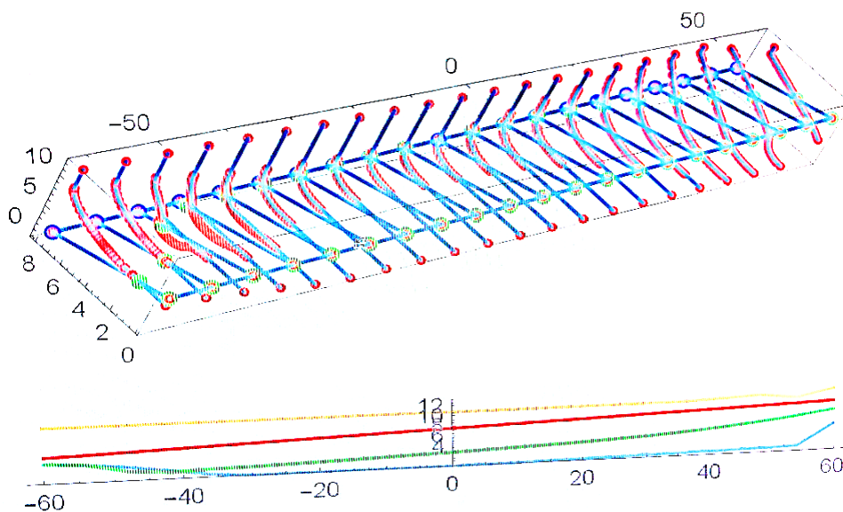
Рисунок 6 – Пространственная модель шпангоутной сетки с плоскостью ватерлинии и соответствующие проекции корпуса с ватерлинией по диаметральной плоскости и на борт
