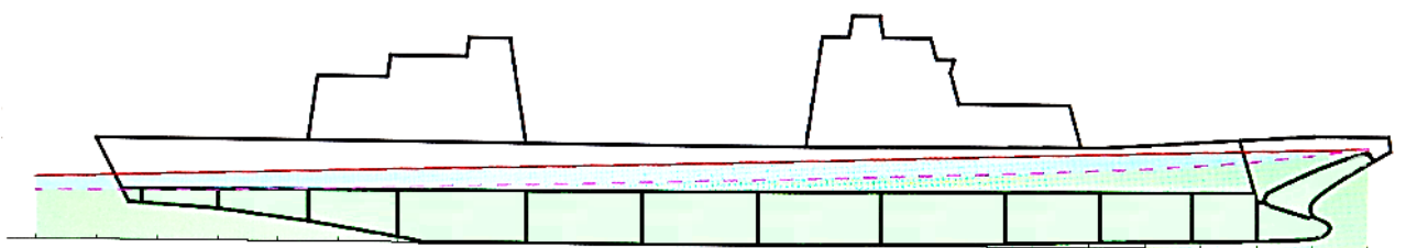
Рисунок 5 – Продольный разрез со схемой непроницаемых отсеков, с ватерлиниями по диаметральной плоскости и проекция ватерлинии на борт
