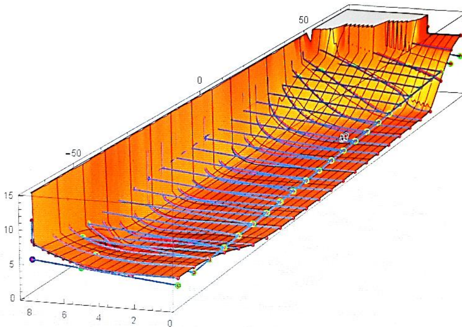
Рисунок 7 – Пространственная модель корпуса с пространственной плоскостью ватерлинии с учетом крена и дифферента
