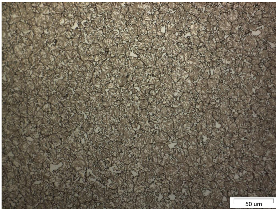
Рисунок 3 - Микроструктура сердцевины образца из стали P18 \times 500
