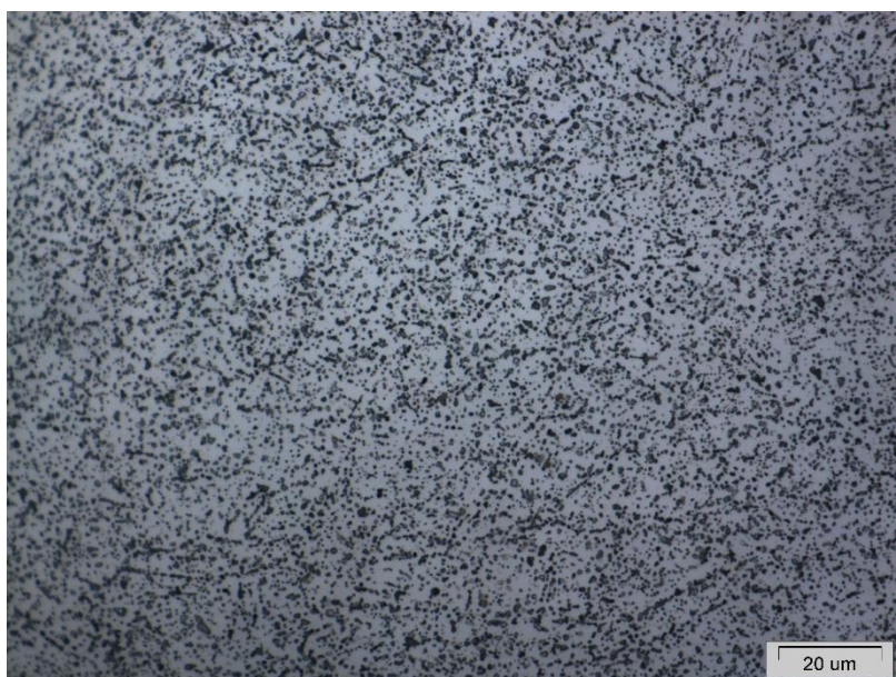
Рисунок 1 - Микроструктура стали со сверхравновесным содержанием азота после ротационной ковки (а) и поперечно-винтовой прокатки (б) с последующим отжигом
