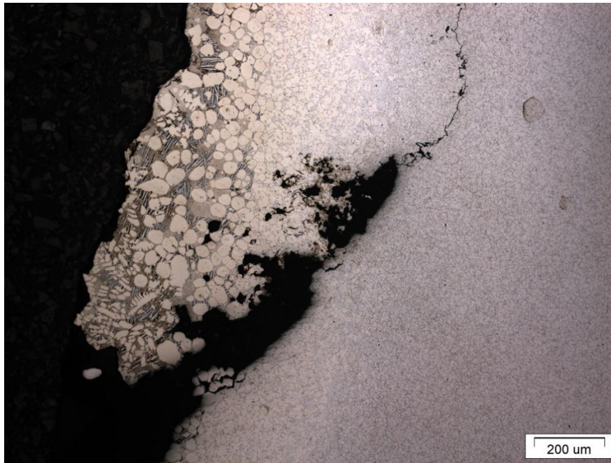
Рисунок 2 - Микроструктура поверхности образца из стали P18 в области дефекта (оплавления) \times 100
