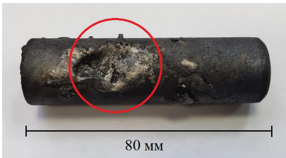
Рисунок 1 - Вид поверхности ролика после термической обработки (заковки с последующим охлаждением в масле) в твердом карбюризаторе
