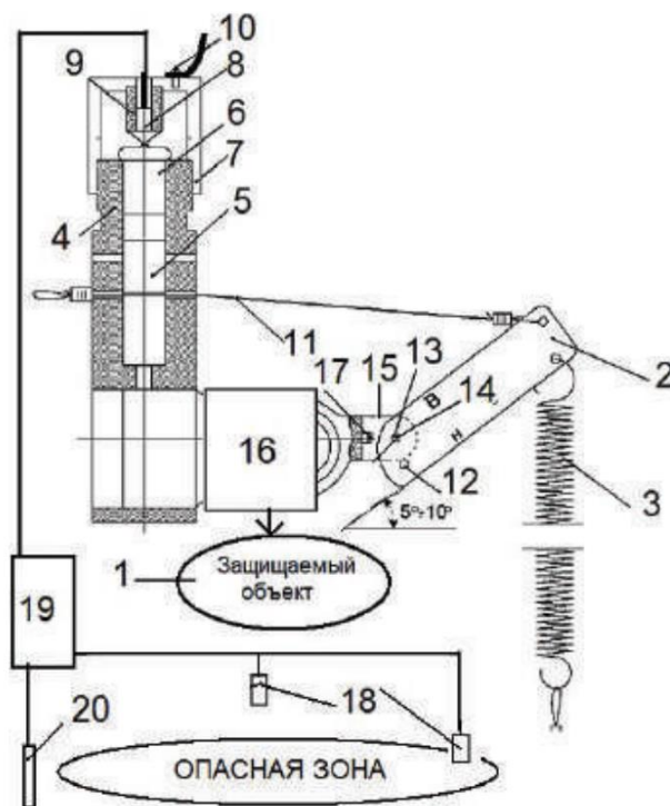
Рисунок 1 - Принципиальная схема автоматического предохранительного устройства систем безопасности в чрезвычайных ситуациях
