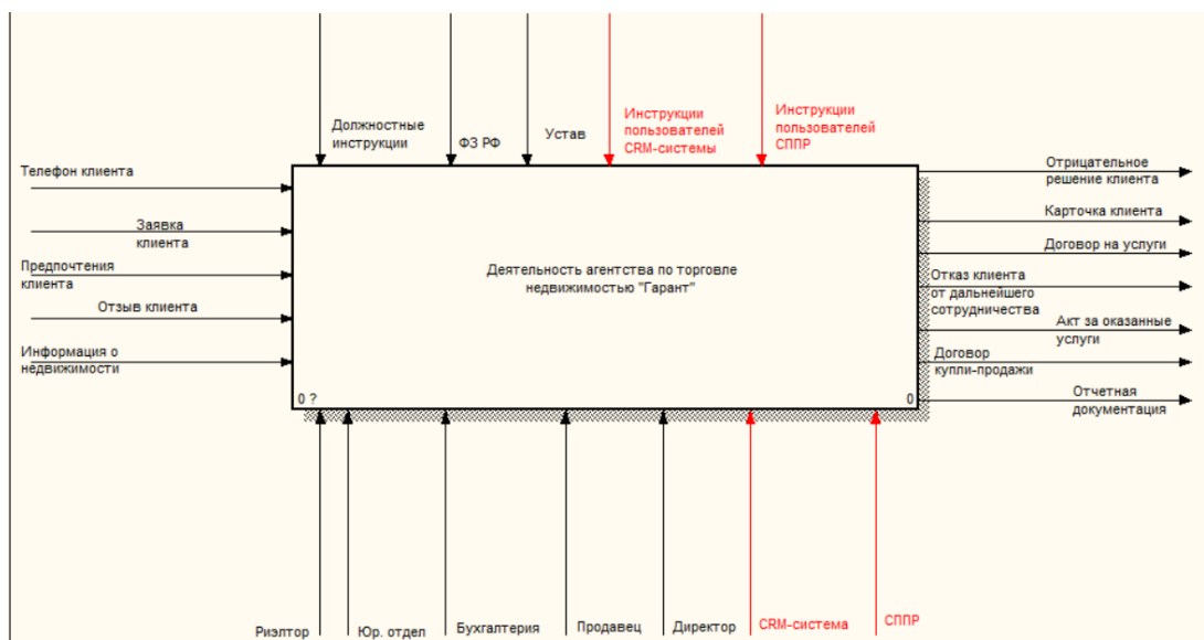
Рисунок 1 – Контекстная диаграмма
