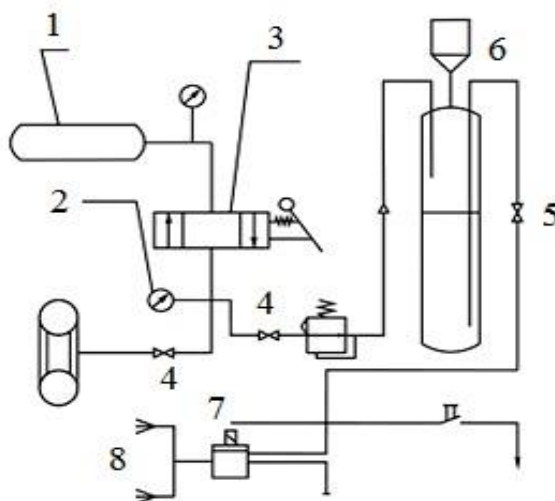
Рисунок 1 - Устройство для пуска двигателя при низких температурах
