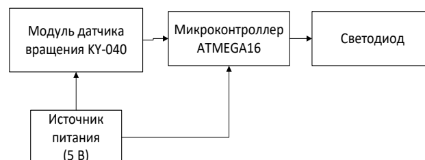
Рисунок 2 - Структурная схема разрабатываемого устройства
