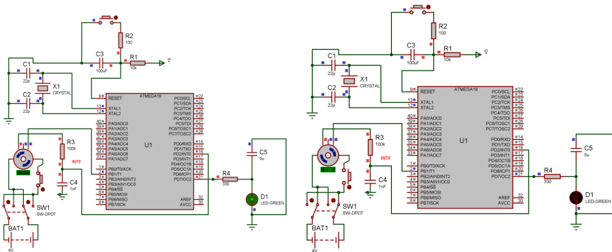
Рисунок 7 - Результат вращения по часовой (слева) и против часовой (справа) стрелки
