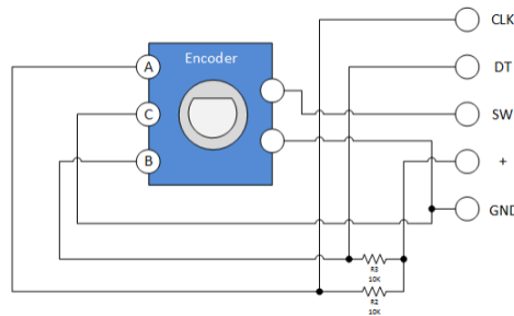
Рисунок 1 — Структура датчика вращения KY-040
