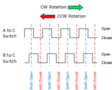
Рисунок 4 - Диаграммы работы датчика вращения KY-040
