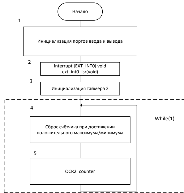
Рисунок 6 - Блок-схема алгоритма ШИМ-регулирования яркости свечения светодиода
