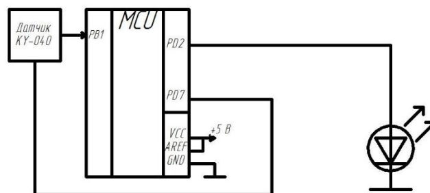
Рисунок 3 - Функциональная схема измерителя разрабатываемого устройства
