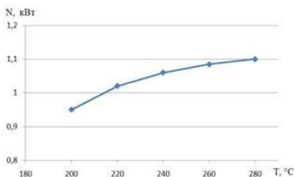
Рисунок 2 - Зависимость мощности двигателя от температуры термической обработки древесного топлива
