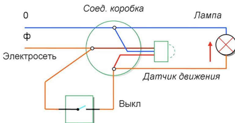
Рис. 1. Схема датчика
