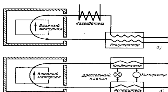
Рисунок 1 - Экспериментальные исследования процесса конвективной сушки пилломатериалов с использованием теплового насоса
