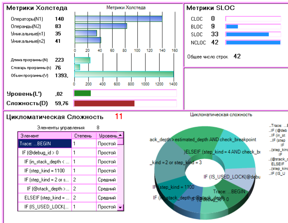
Рис. 7. Аналитический отчет сложности по выбранной процедуре из списка
