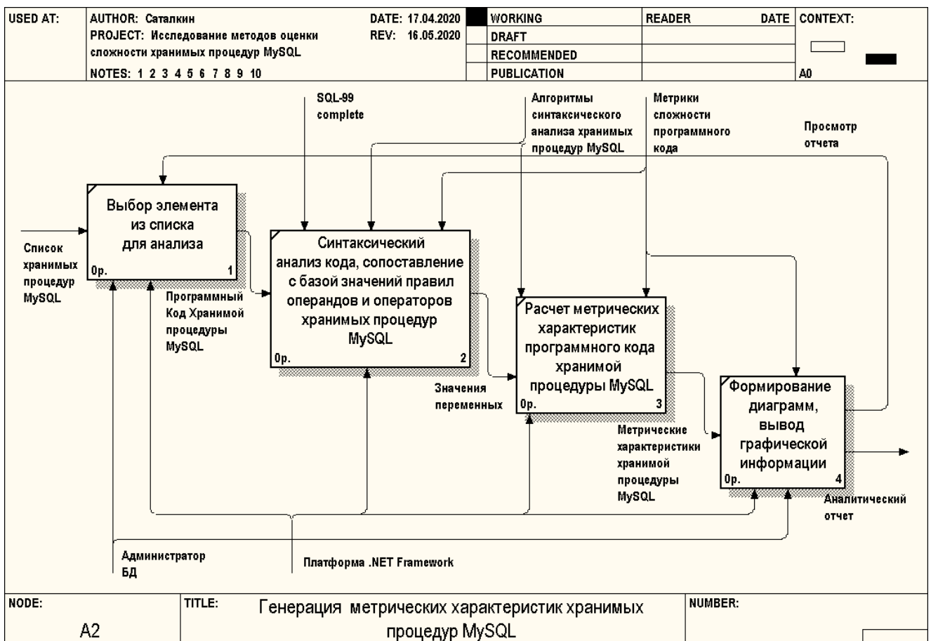
Рисунок 1. Диаграмма IDEF0 декомпозиция процесса генерации метрических характеристик
