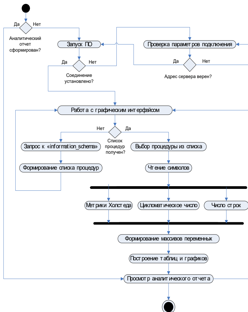
Рисунок 2 – Общая диаграмма активности системы
