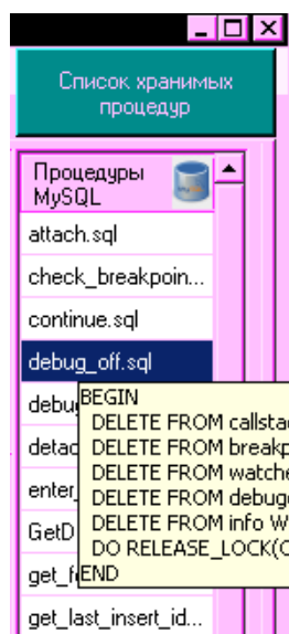
Рис. 5. Фрагмент списка хранимых процедур
