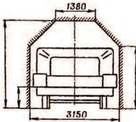
Рис. 1. Железнодорожный габарит 02 - Т
