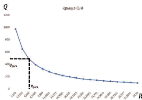
Рисунок 3. Теплопотери крыши
