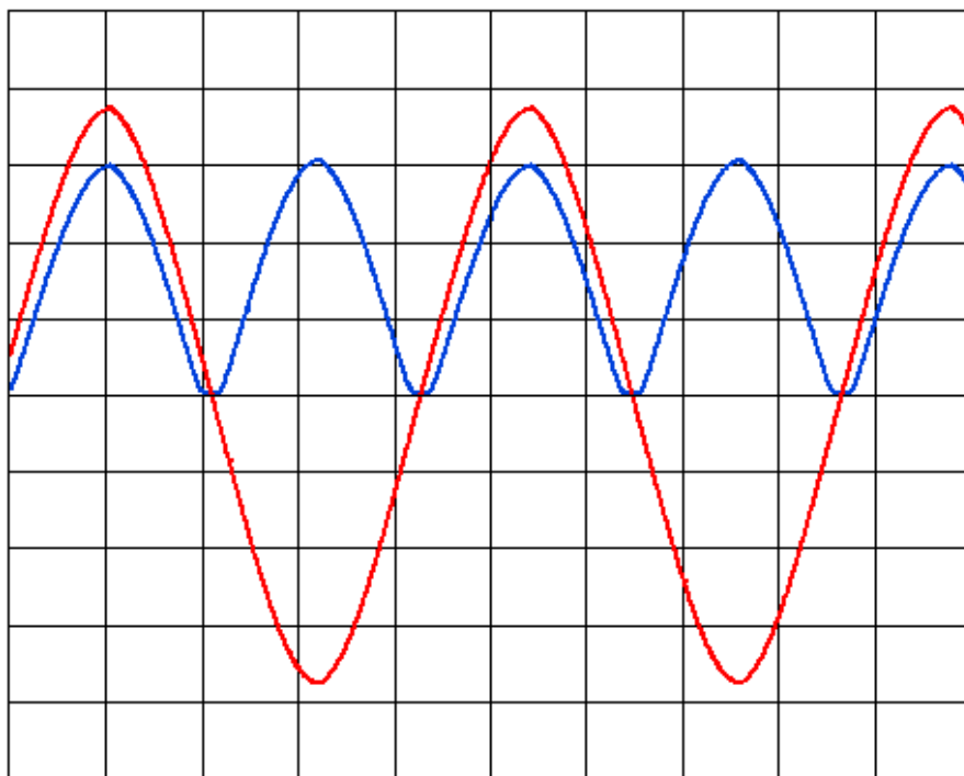
Рисунок 2. График входного и выходного напряжения
