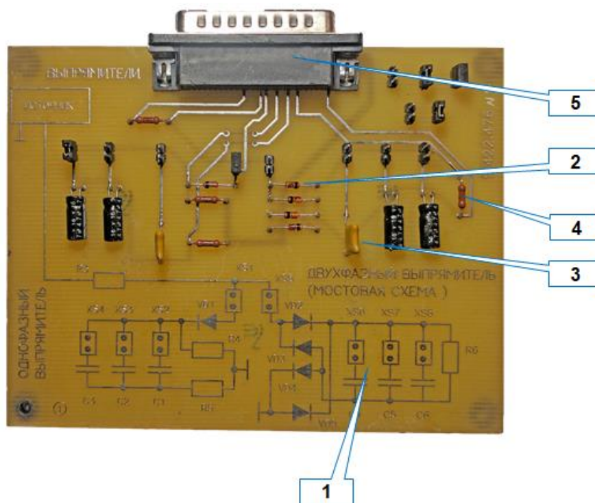
Рисунок 1. Лабораторная плата «Выпрямители»
