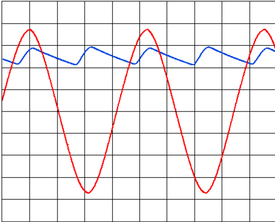
Рисунок 4. Входное и сглаженное напряжение на нагрузке
