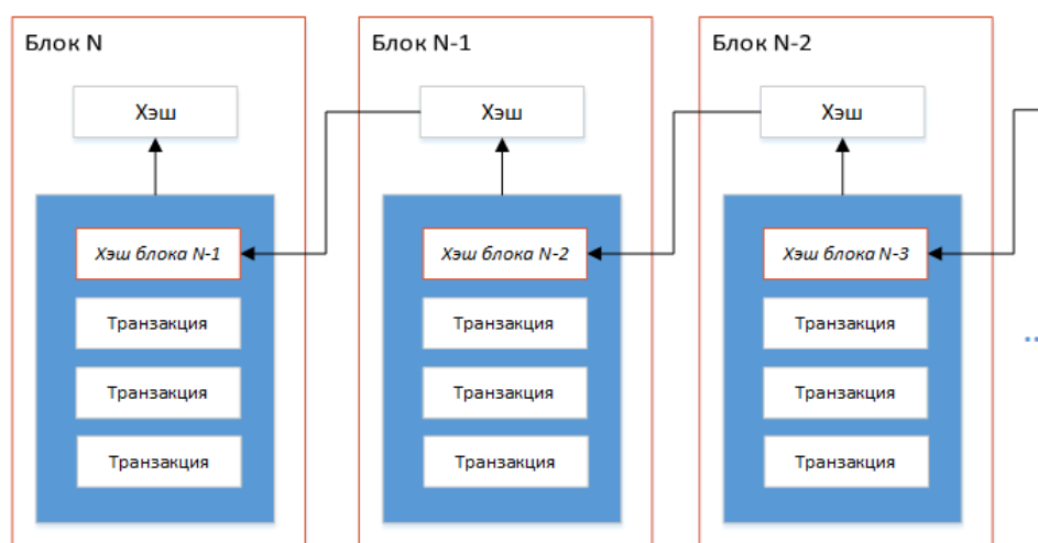
Рис. 2 Пример цепочки последовательных блоков
